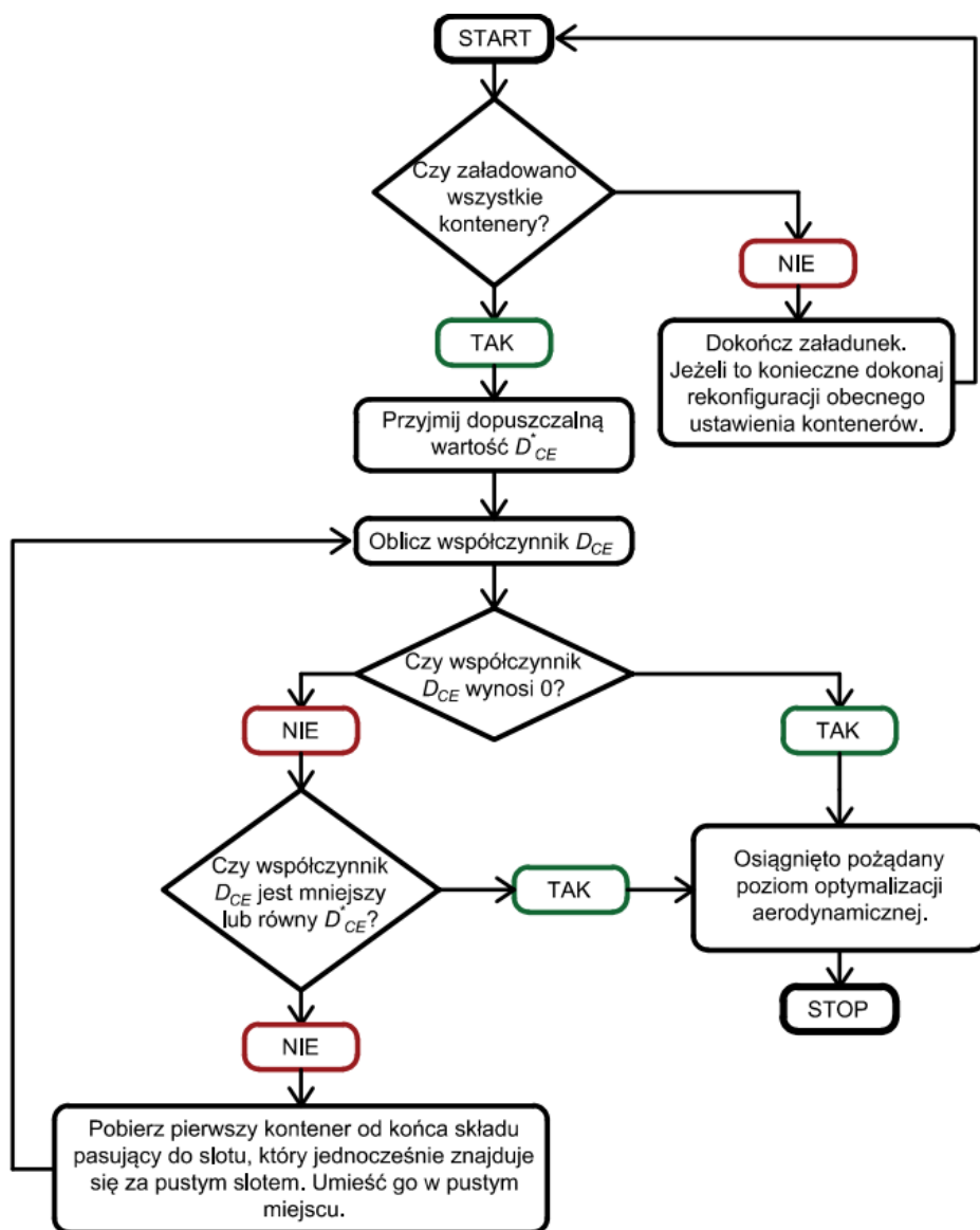
Rys. 5. Przykład algorytmu optymalizacyjnego aerodynamiki pociągu intermodalnego podczas załadunku. Źródło: opracowanie własne
